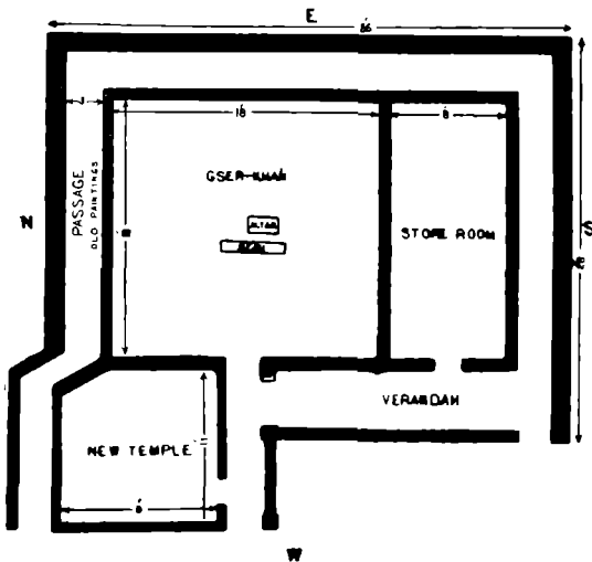
GSER-KHAÑ TEMPLE SKETCH PLAN
